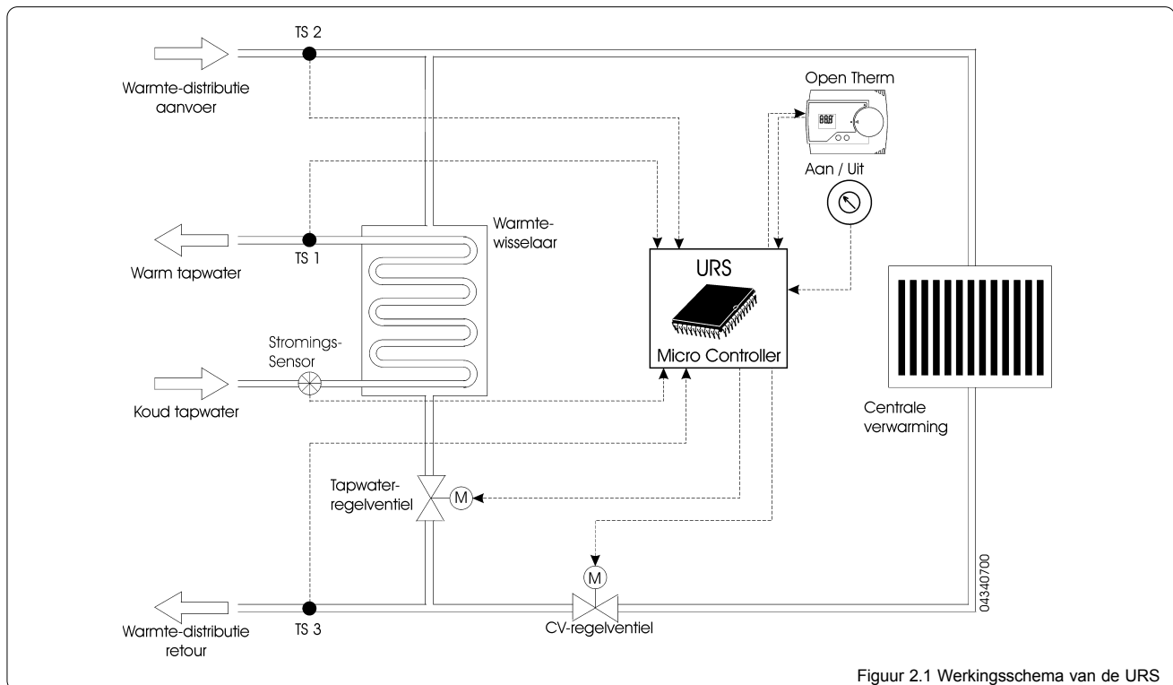
Figuur 2.1 Werkingsschema van de URS
