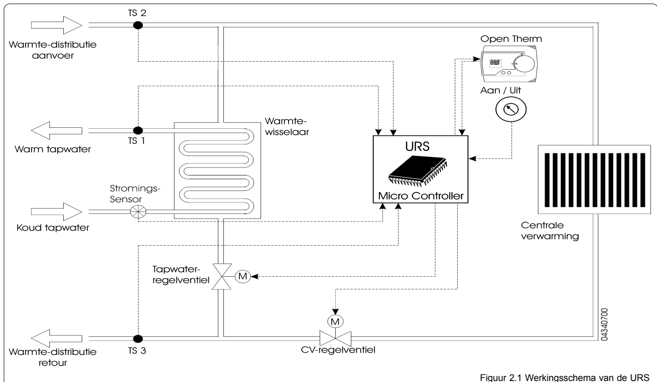
Figuur 2.1 Werkingsschema van de URS
