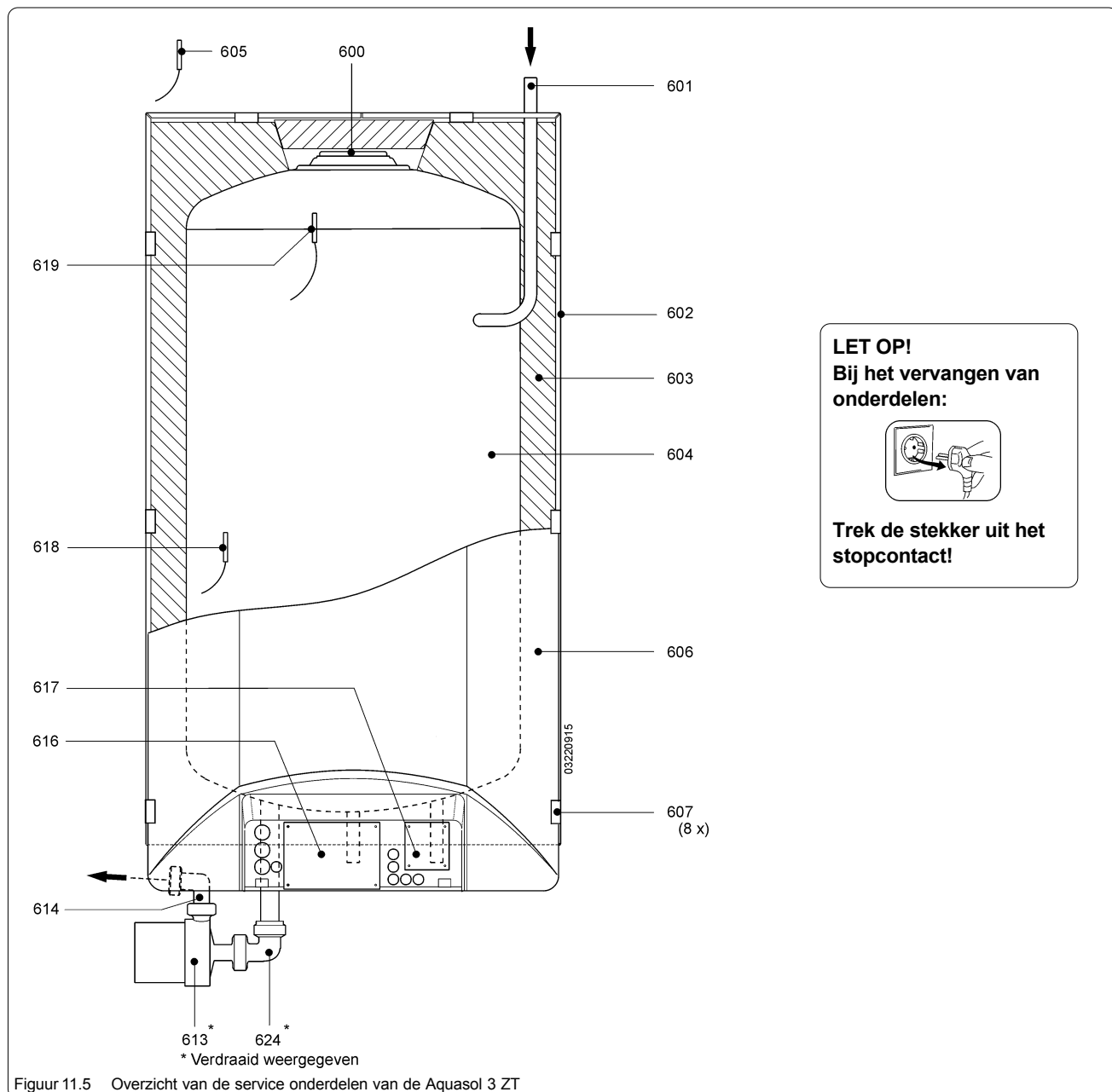
Figuur 11.5 Overzicht van de service onderdelen van de Aquasol 3 ZT
