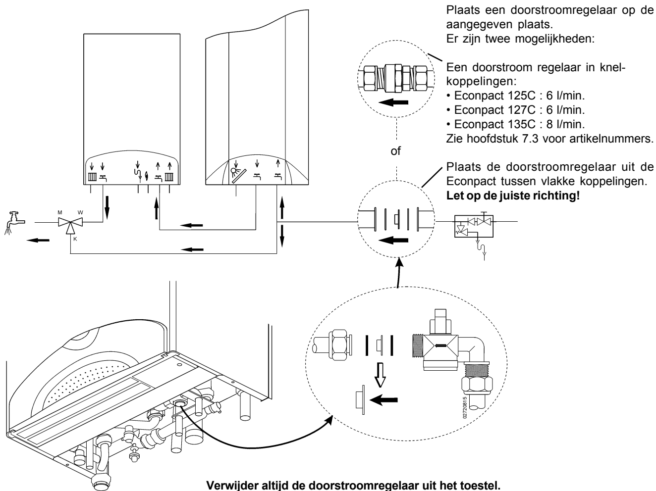
Figuur 8.2 Tapwaterzijdige aansluiting van de AquaSol 3 ZT op de Econcompact 125C, 127C of 135C
