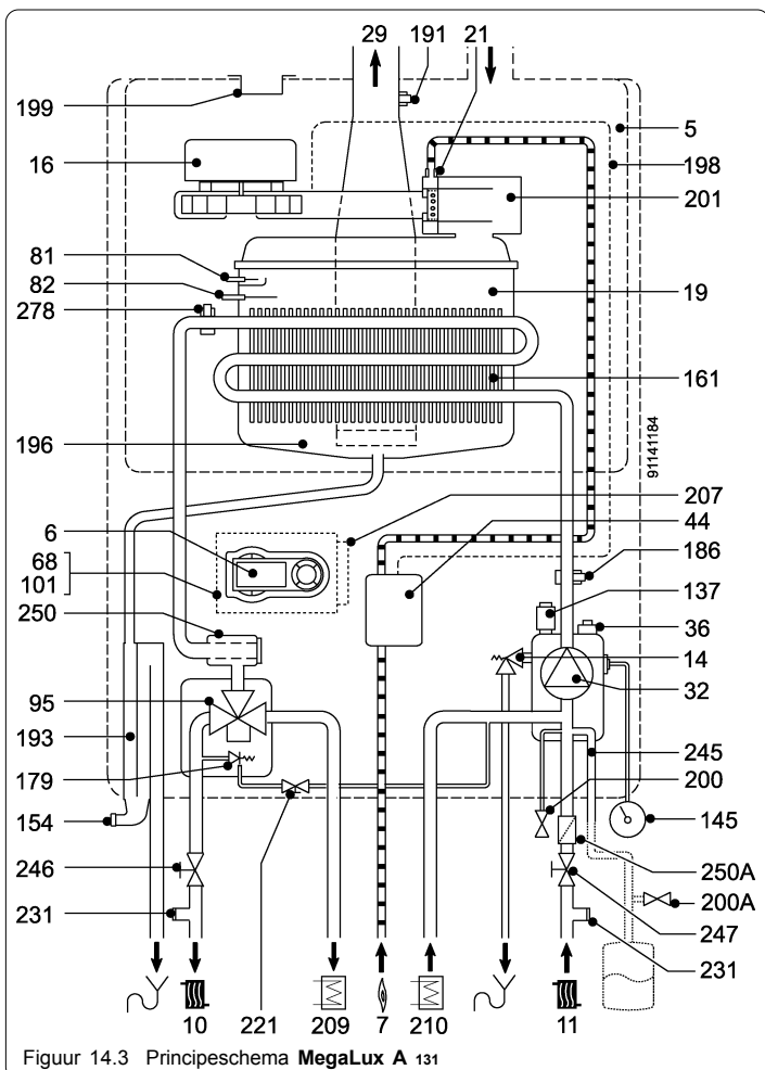
Figuur 14.3 Principeschema MegaLux A 131
