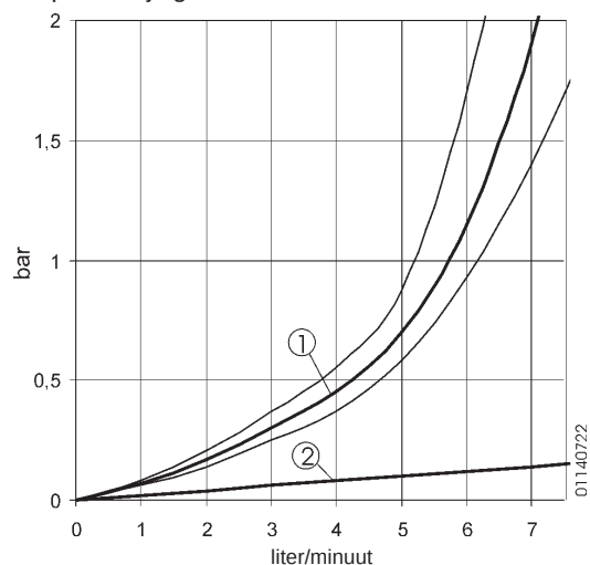
Tapwaterzijdig drukverlies ECONPACT 27C
