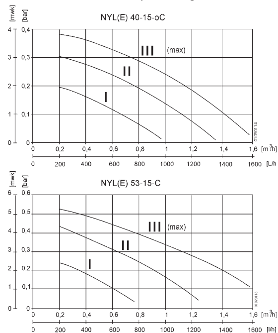
De externe beschikbare opvoerhoogte
