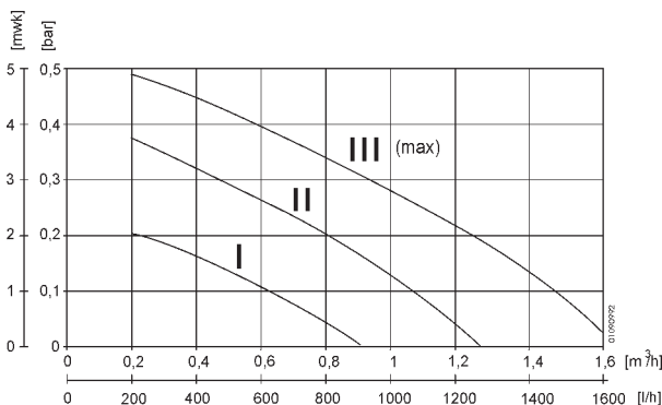
De externe beschikbare opvoerhoogte bij de ECONPACT 27/35 A/C.
