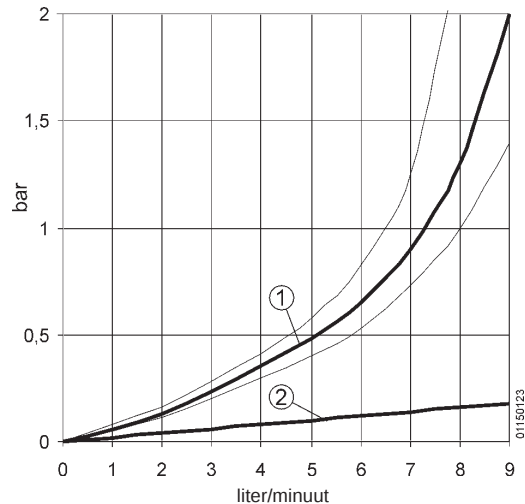
Tapwaterzijdig drukverlies ECONPACT 35C
