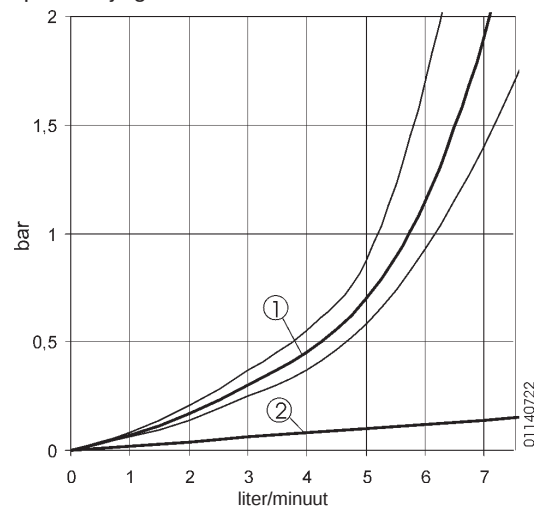
Tapwaterzijdig drukverlies ECONPACT 125/127/225C
