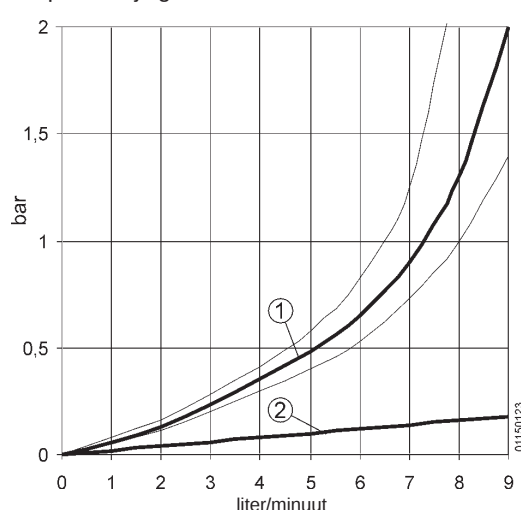
Tapwaterzijdig drukverlies ECONPACT 135/235C
