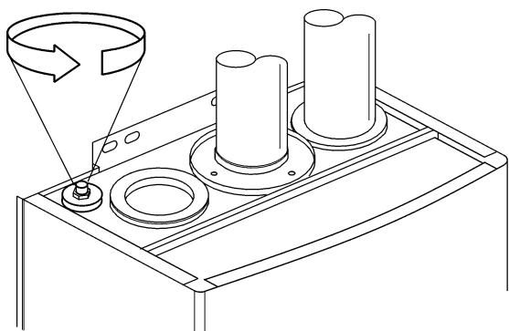
Figuur 10.2 De automatische ontluchter
