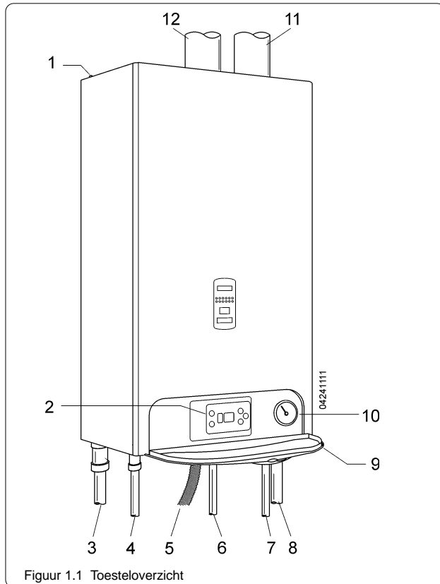
Figuur 1.1 Toesteloverzicht
